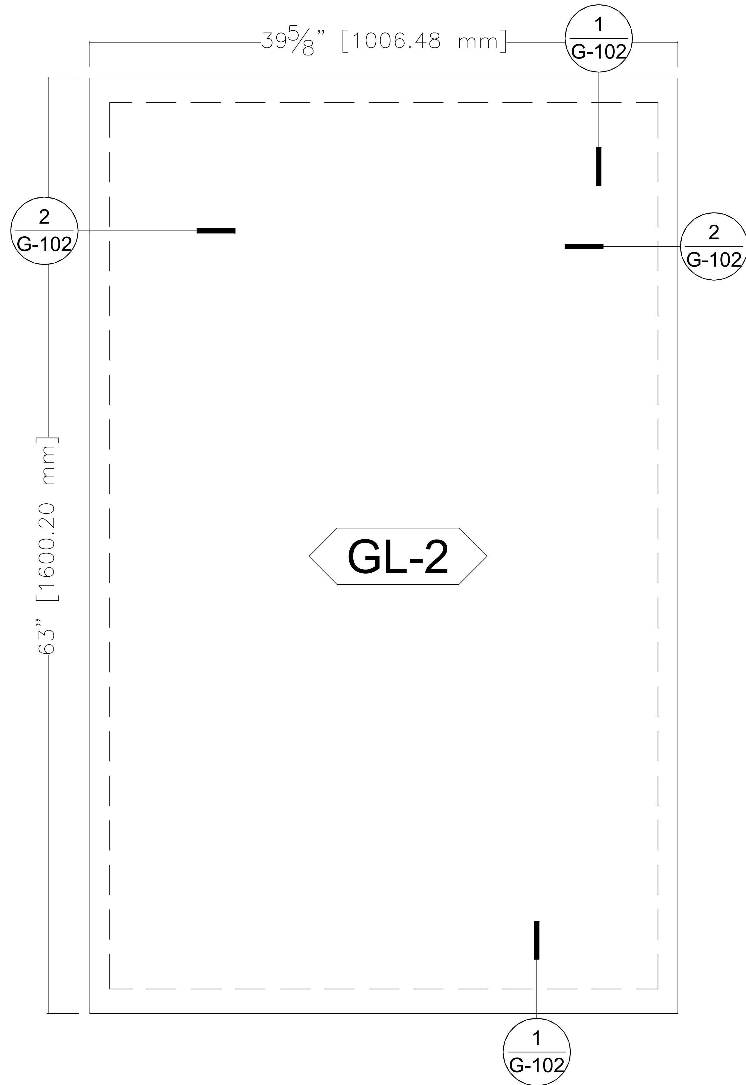
1 PLAN - GLASS UNIT A GL-2 - QTY 1 Scale: 3"=1'-0"
